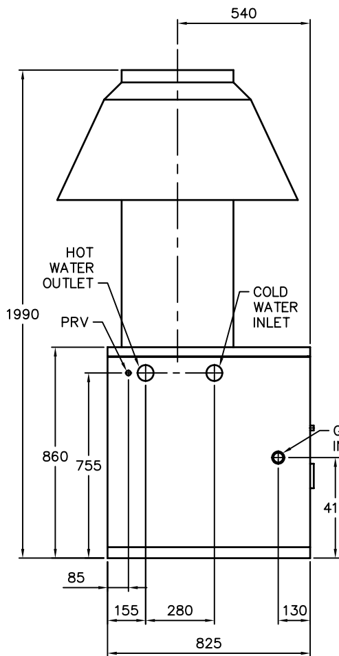
LEFT SIDE
