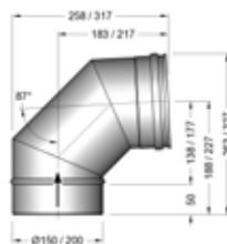
87° Elbow
