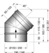
45° Elbow
